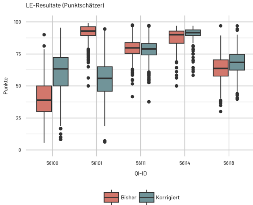
Abbildung 1: Boxplots mit Median, Minimum und Maximum der LE-Ergebnisse (Punktschätzer) der bisherigen und korrigierten Berechnung im Vergleich
